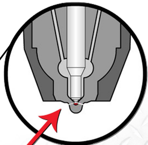
ECOTIP ® Nozzle
